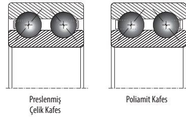
Şekil 2. Kafes tipleri: çift sıra
