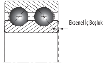
Şekil 13. Çift sıra aksel boşluk.
